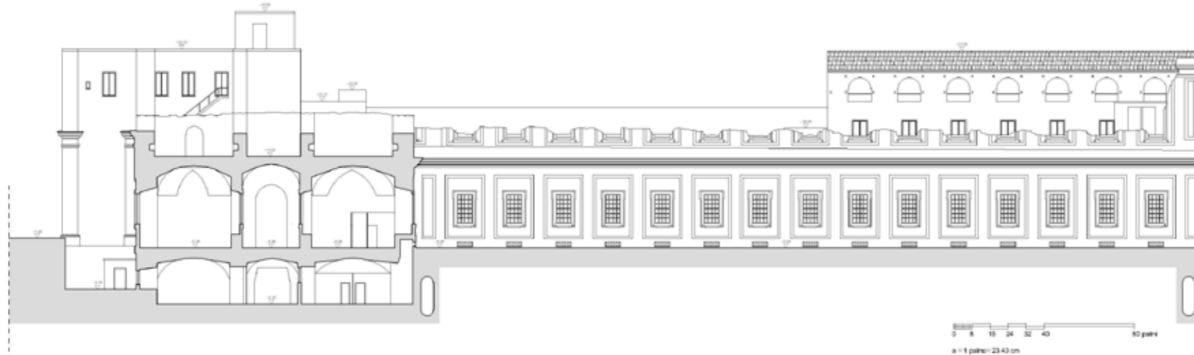
Extrait de coupe-façade de l'état des lieux
