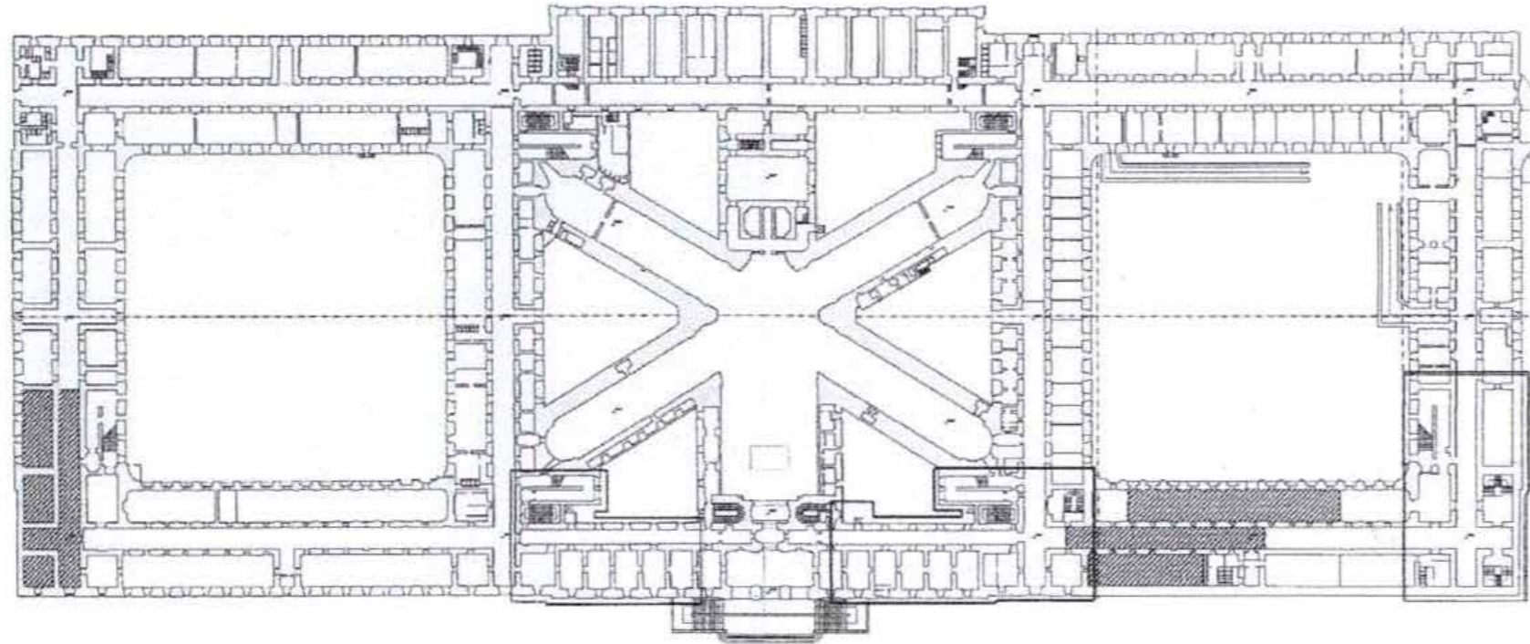
Plan de l'état des lieux
